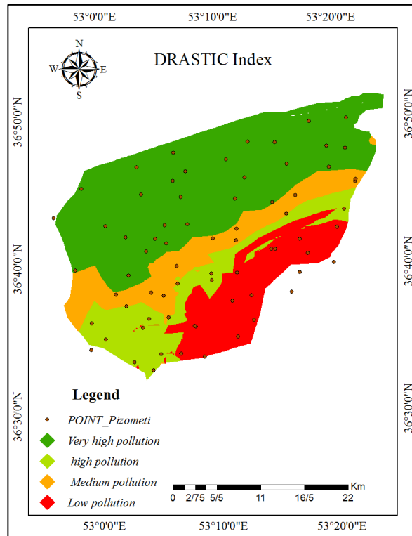
شکل (3): نقشه همپوشانی مدل DRASTIC بر اساس هفت پارمتر موثر در ارزیابی آلودگی دشت نکارود
