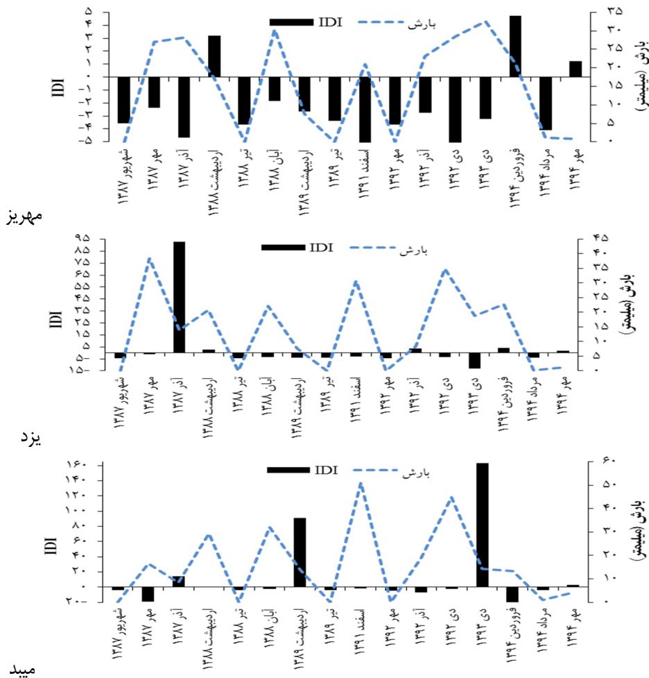
شکل (۹): مقایسه بین میانگین نمایه تأثیر خشکسالی (IDI) با بارندگی در محدوده مهریز، میبد و یزد
