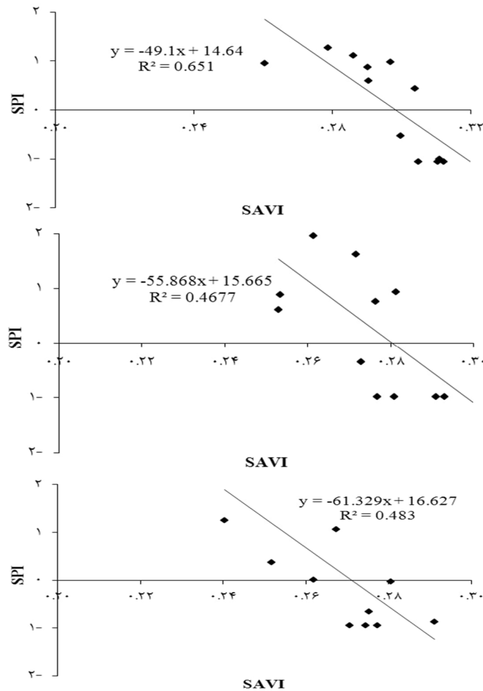
شکل (۷): رابطه بین شاخص پوشش گیاهی SAVI با SPI همان ماه در مراتع محدوده مهریز، یزد و میبد
