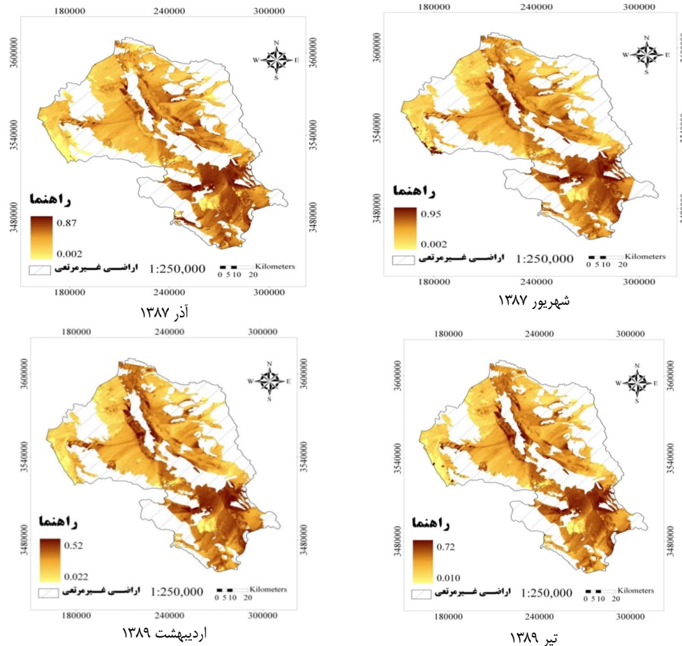
شکل (۶): نقشه شاخص SAVI در دوره‌های مختلف در منطقه مورد بررسی
