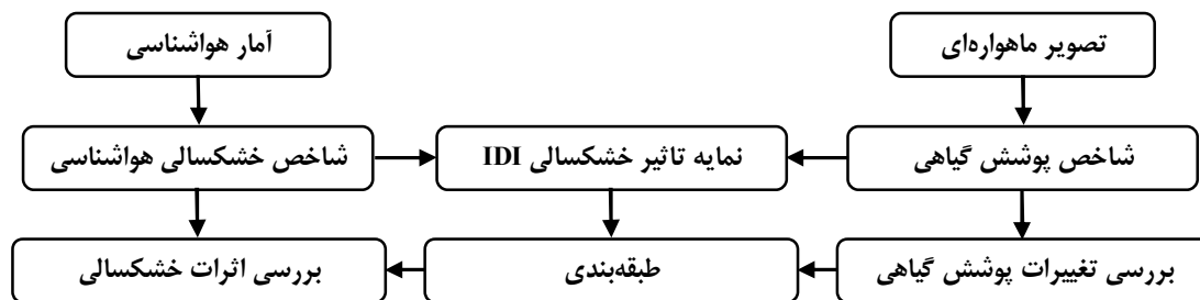
شکل (۳): روند نمای روش کار
