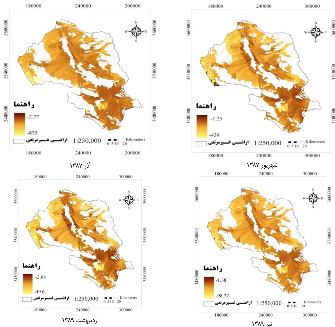
شکل (۸): نمایه تأثیر خشک‌سالی (SWDI) در مراتع دشت یزد- اردکان در برخی ماه‌ها
